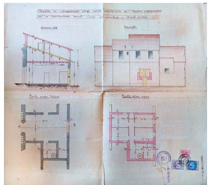
Disegno estratto dall'istanza n. 22626 del 10 giugno 1919, conservata presso l'Archivio Storico del Comune di Livorno
